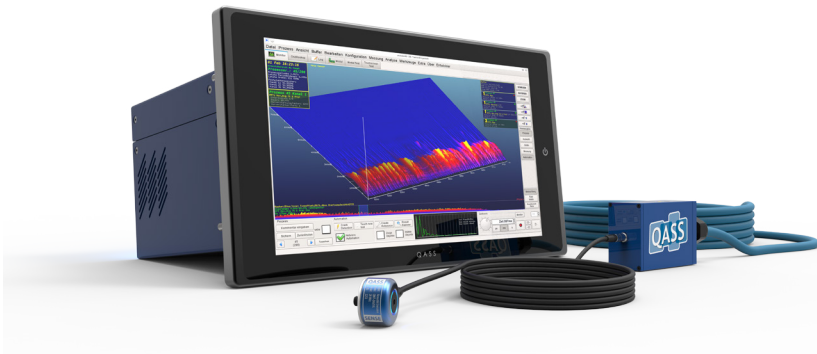
Abb. 1: Optimizer4D in der Gehäusevariante für den Schaltschrank, mit Vorverstärker und HFIM-Sensoren.
